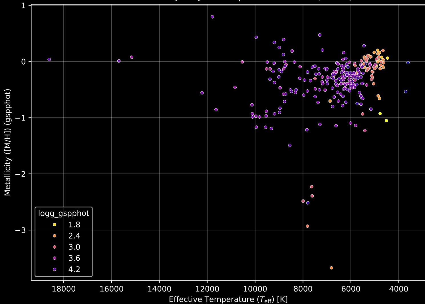
GALAH DR4 Field: [9473] Stellar Population Parameters (n= 276)
