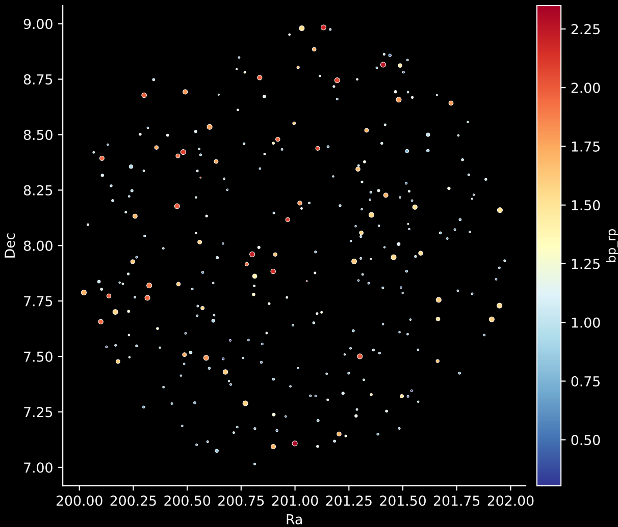
GALAH DR4 Field: [9473] Stars: 276
